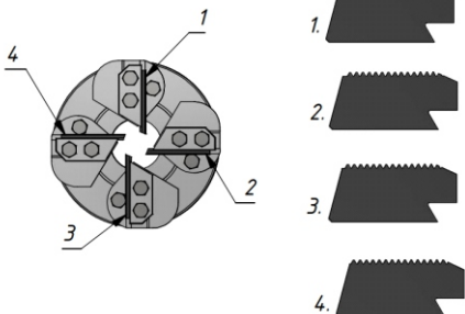
Рис.1 Резьбонарезная головка
